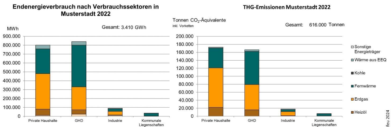
Abbildung 19: Exemplarische Darstellung der Energie- und THG-Bilanz für Wärme nach Sektoren für eine Musterstadt. Quelle: Darstellung ifeu
