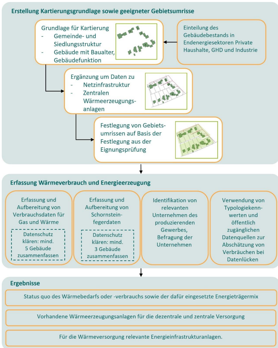
Abbildung 11: Übersicht zur Vorgehensweise in der Bestandsanalyse. Quelle: Darstellung ifeu
