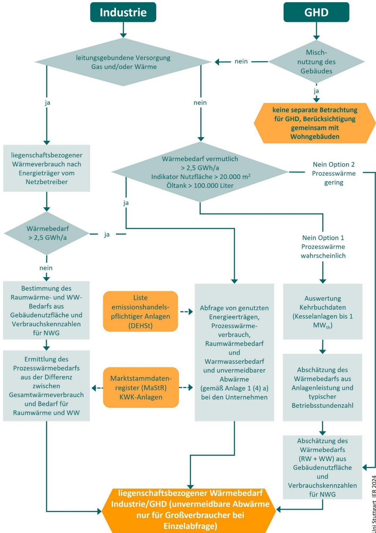
Abbildung 16: Darstellung der Vorgehensweise im Bereich GHD und Industrie zur Ermittlung des Wärmebedarfs und der unvermeidbaren Abwärme. Quelle: Darstellung Universität Stuttgart IER
