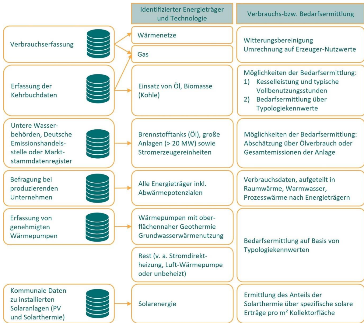
Abbildung 14: Darstellung der Wärmeverbrauchs- bzw. -bedarfsermittlung je nach Energieträger und Wärmeversorgungstechnologien und dazugehörigen Datenquellen. Quelle: Darstellung ifeu
